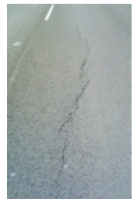
Longitudinal crack
